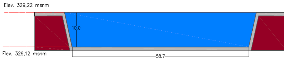
Figura 31. Vista frontal del vertedor cipolletti
