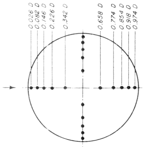
Figura 3.1 Puntos de medición de velocidad del aire.
