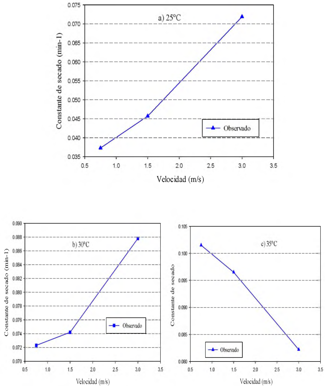
Figura 2.14 Efecto de la velocidad sobre la constante de secado en semilla de papaya para las tres temperaturas.
