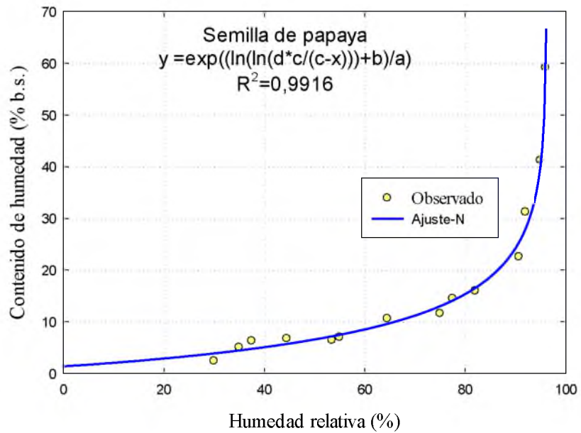
Figura 2.18. Nuevo modelo matemático de equilibrio para la semilla de papaya Pococi.
